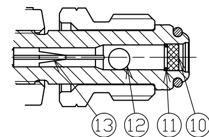
B 詳細(1:1)
